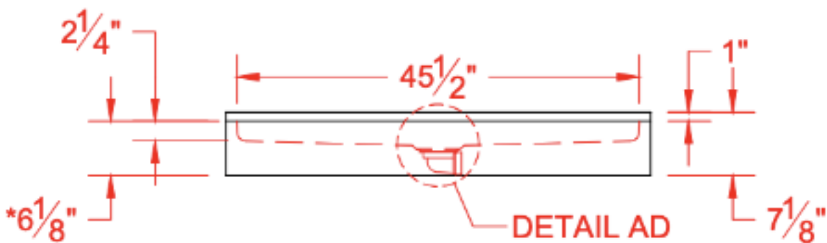
FRONT ELEVATION - SCALE: \frac{3}{8} " = 1'-0"
